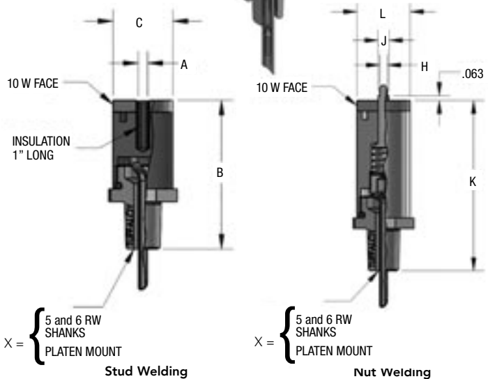
Stud Welding
